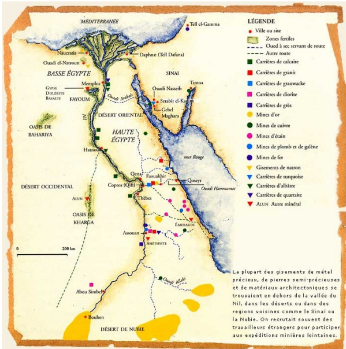
Les ressources minérales de l'Égypte ancienne. Carte tirée de l'ouvrage "Au cœur de l'Égypte ancienne" Larousse-Bordas. Paris 1997.
